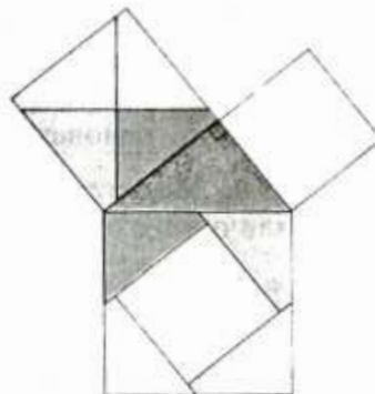
Питагорина теорема
